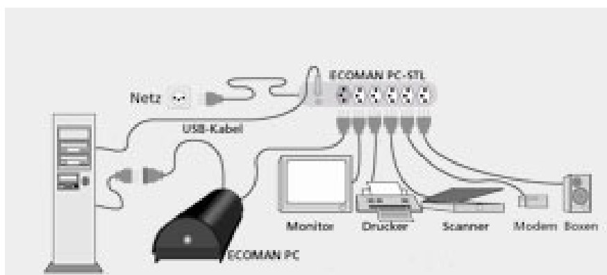
Figur 6: Schematische Installation von Ecoman PC-STL und Ecoman PC
